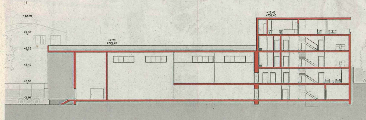
Diese Zeichnung skizziert, wie das neue Gebäude von Koco Motion und Koco Automotive aussehen soll. Auf der rechten Seite des Gebäudes ist der Bürotrakt zu sehen.
